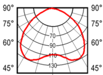
Кривые силы света светильника
